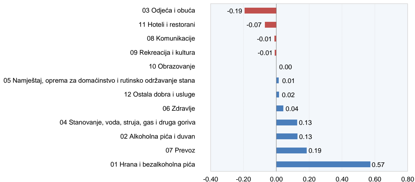
Grafik 2. Uticaj pojedinačnih oblasti na godišnju stopu inflacije (u procentnim poenima), mart 2021.
