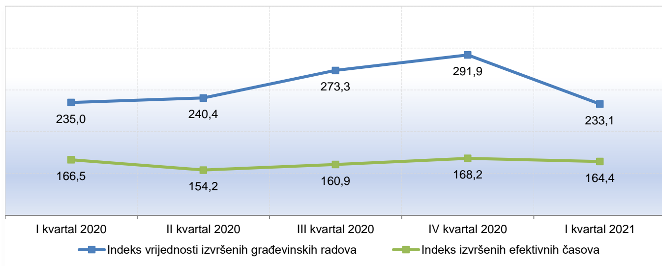
Grafik 1. Indeksi vrijednosti građevinskih radova i izvršenih efektivnih časova, 2015=100 1
