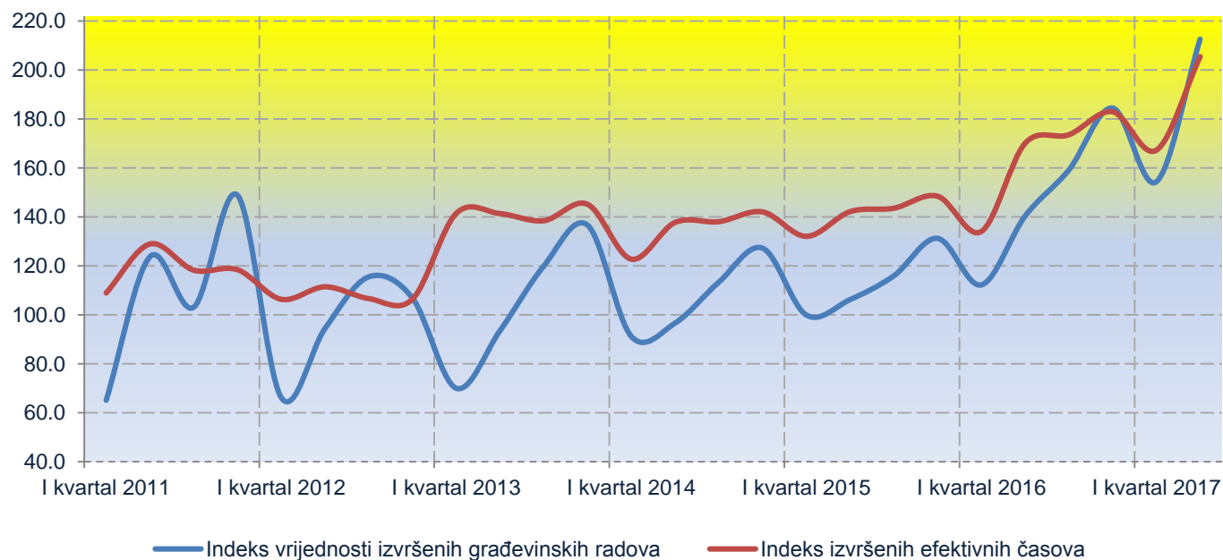
Grafik 1. Indeksi vrijednosti građevinskih radova i izvršenih efektivnih časova, 2010=100
